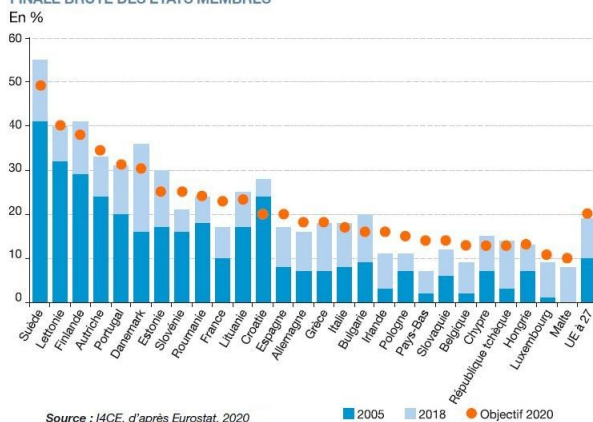
PART DES ÉNERGIES RENOUVELABLES DANS LA CONSOMMATION ÉNERGÉTIQUE FINALE BRUTE DES ÉTATS MEMBRES
